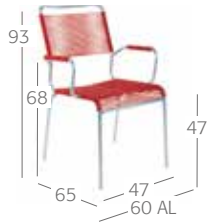
«Spaghetti»-Bespannung | Arm- lehnen Look «Spaghetti» | accoudoirs «Spaghetti» design | arm rests 28041
