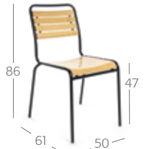
Schweizer Holzplatten Lattes en bois suisse Swiss wooden slats 21030
