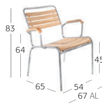
Sessel | Schw. Holzlatten | Armlehnen Siège | lattes en bois suisse | accoudoirs Lounge chair | Swiss wooden slats | arm rests 21037
