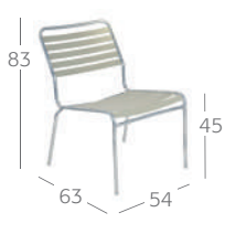
Sessel | Latten Siège | Lattes Lounge chair | slats 21100
